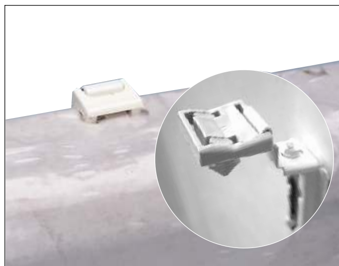
Art.-Nr. 1-002512 Art.-Bez. Vormontageadapter für Folienmontage
