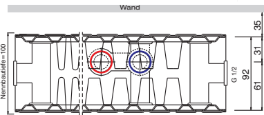
Typ 22 plus / 22 Bautiefe 100 mm
