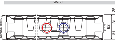
Typ 21 Bautiefe 70 mm
