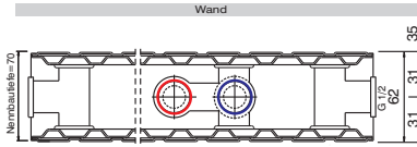
Typ 20 Bautiefe 70 mm
