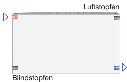
Anschlussvariante "Kompakt", Vorlauf / Rücklauf wechselseitig
