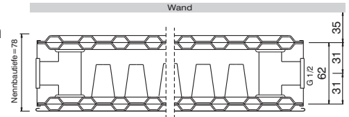
Typ 21 Bautiefe 78 mm
