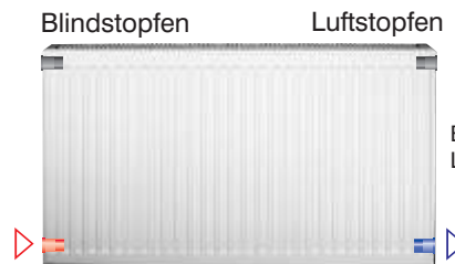
Anschlussvariante "Kompakt", Vorlauf und Rücklauf reitend
