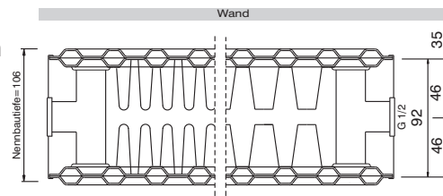
Typ 22 plus / 22 Bautiefe 106 mm
