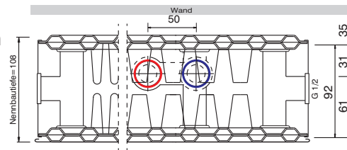
Typ 22 plus / 22 Bautiefe 108 mm
