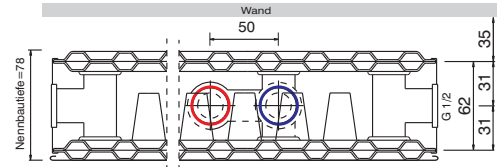
Typ 21 Bautiefe 78 mm
