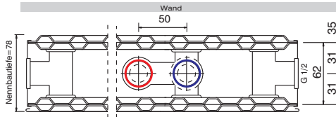
Typ 20 Bautiefe 78 mm
