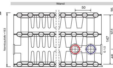
Typ 33 plus / 33 Bautiefe 163 mm
