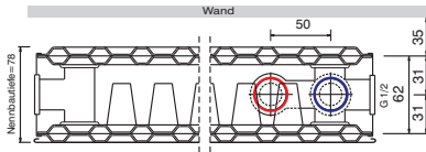
Typ 21 Bautiefe 78 mm
