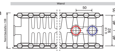
Typ 22 plus / 22 Bautiefe 108 mm
