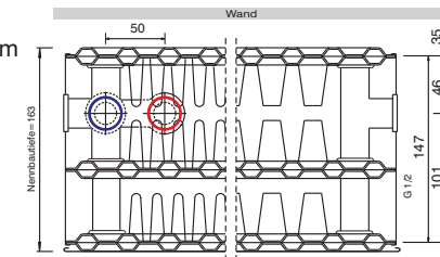
Anschlussvariante "Ventil", Vorlauf / Rücklauf von unten
