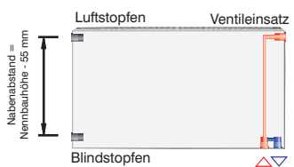
Anschlussvariante "Kompakt", Vorlauf / Rücklauf gleichseitig
