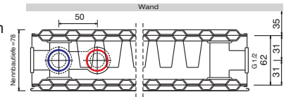
Typ 21 Bautiefe 78 mm
