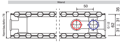
Typ 20 Bautiefe 78 mm
