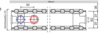
Typ 20 Bautiefe 78 mm
