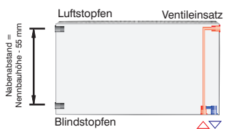
Anschlussvariante "Kompakt", Vorlauf / Rücklauf gleichseitig
