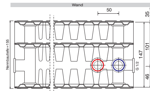
Typ 33 plus / 33 Bautiefe 155 mm
