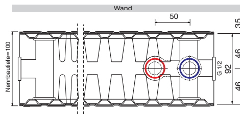
Typ 22 plus / 22 Bautiefe 100 mm
